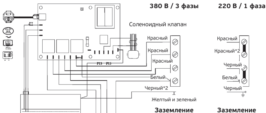
Рисунок 1. Схема подключения парогенератора
